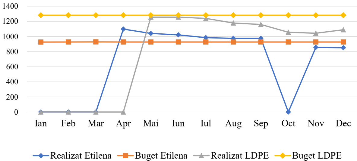
Evolutia lunara a costului pentru etilena / pretul de vanzare pentru LDPE comparativ cu programul (USD/tona) pentru anul 2025
